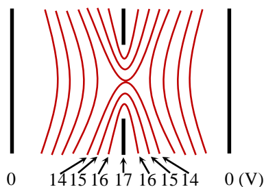
Σχήμα Π33.5. Το δυναμικό στις οπές του διάτρητου δίσκου.
