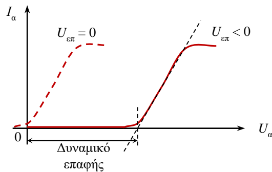
Σχήμα 33.8. Μετατόπιση της καμπύλης ρεύματος-τάσης λόγω αρνητικού δυναμικού επαφής.
