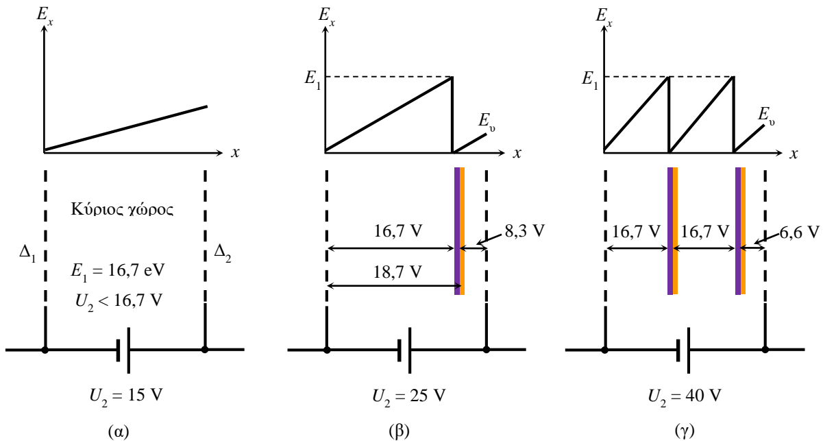
Σχήμα 33.5. Τρεις περιπτώσεις εξέλιξης της κινητικής ενέργειας των ηλεκτρονίων στον κύριο χώρο της λυχνίας.
