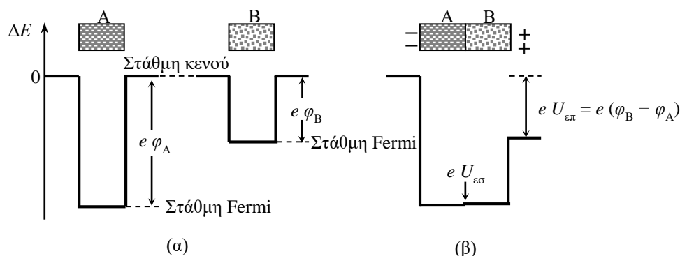
Σχήμα Π33.1. Η δυναμική ενέργεια ενός ηλεκτρονίου μέσα και έξω από τα μέταλλα A και B. (α) Πριν από την επαφή και (β) μετά την επαφή.
