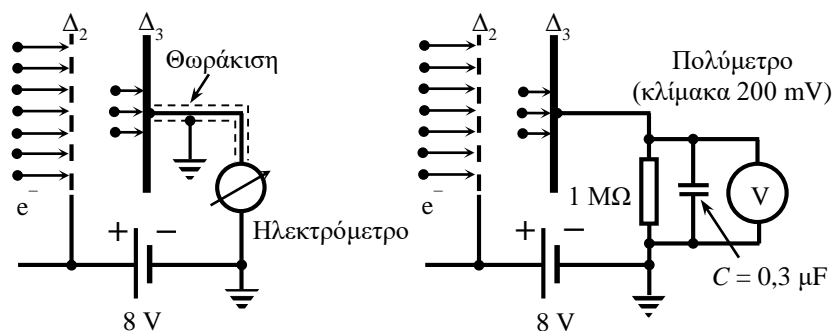
Σχήμα Π33.3. Μέτρηση ασθενούς ρεύματος με χρήση (α) ηλεκτρομέτρου και (β) του αυτοσχέδιου ηλεκτρομέτρου της άσκησης.
