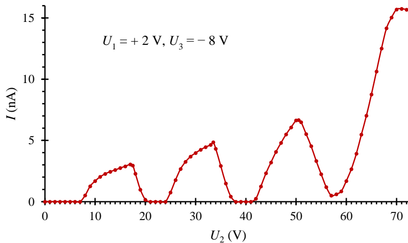
Σχήμα 33.7. Πειραματική καμπύλη ρεύματος-τάσης στη λυχνία Ne.
