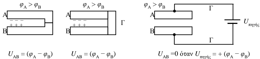
Σχήμα Π33.2. Σύνδεση δύο μετάλλων, Α και Β, με ένα τρίτο μέταλλο, Γ.
