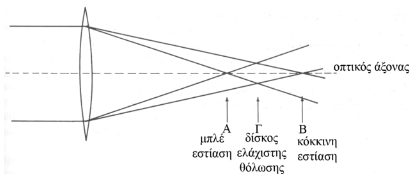
Σχήμα 6. Χρωματική εκτροπή ενός φακού
