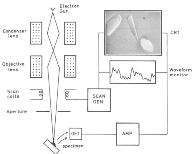
Σχήμα 15. Σχηματικό διάγραμμα SEM και φωτογραφία ενός FEI INSPECT SEM.
