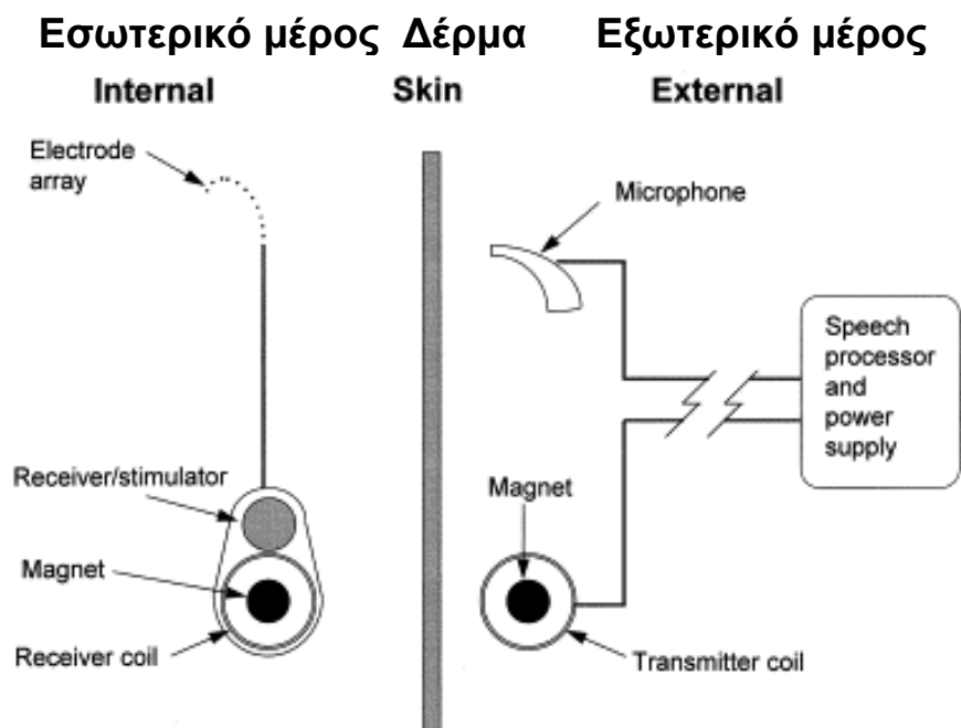
Σχήμα 3. Σχηματικό διάγραμμα των συνιστωσών ενός κοχλιακού εμφυτεύματος.
